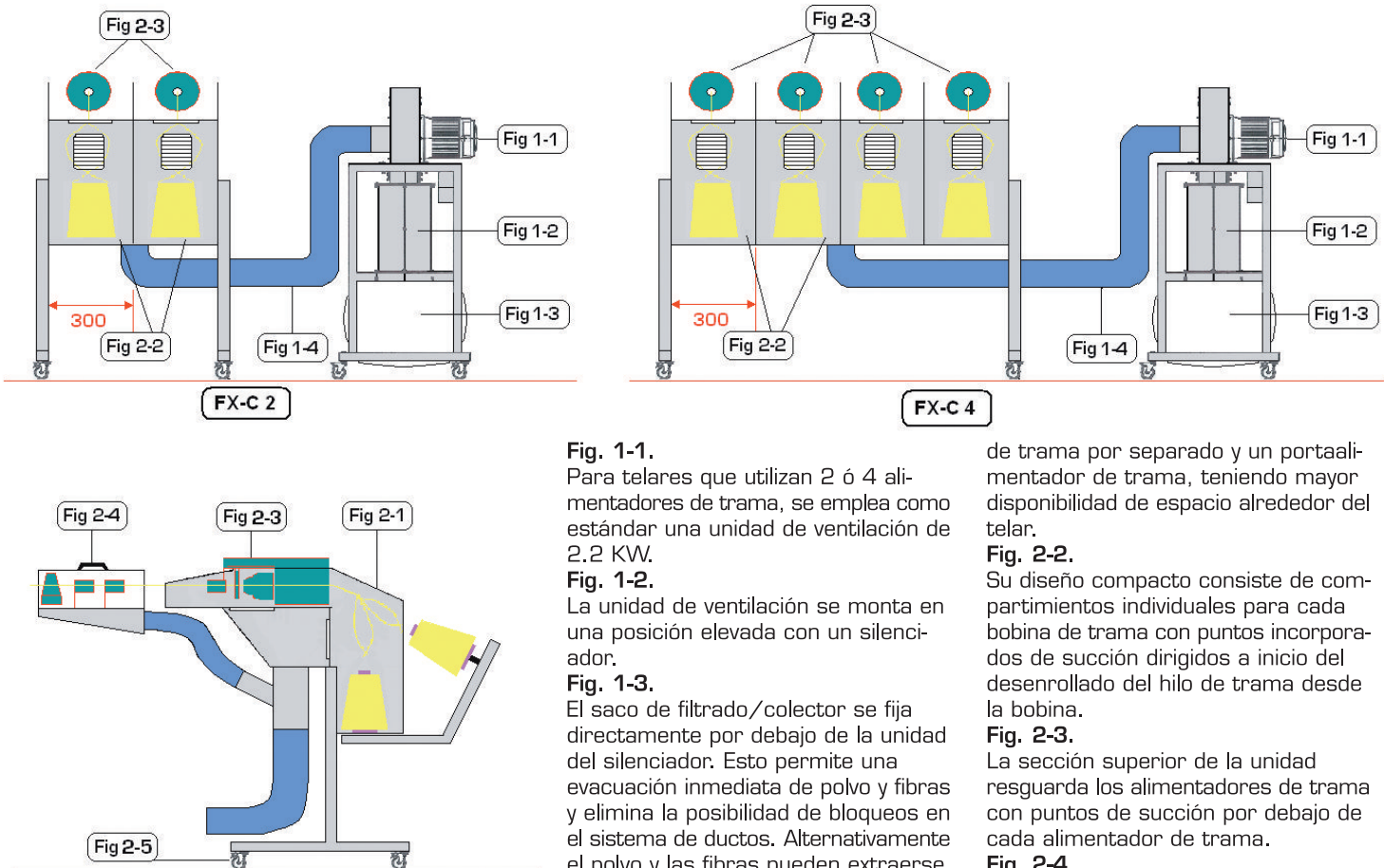
Fig. 2-4. Otros puntos de succión complementarios para dispositivos de tensión de trama y sensores de freno pueden ser dirigidos adicionando una unidad secundaria, colocándola en la parte frontal de la unidad principal.
